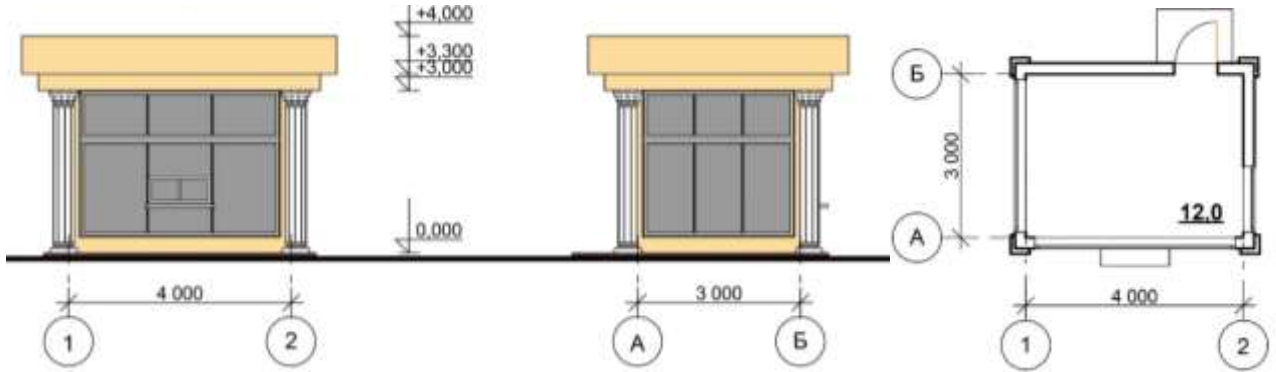
Рис. «Основные параметры места размещения нестационарного торгового объекта для киосков» схемы места размещения нестационарного торгового объекта при островном размещении киоска с тупиковым подходом:
